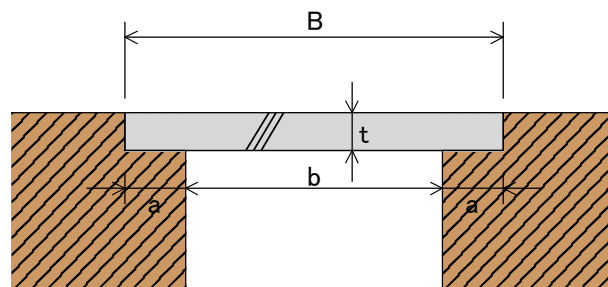
水路幅 b 製品幅 B=2a+b
