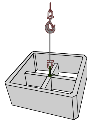
【吊り上げ方法】※ I型II型 共通
