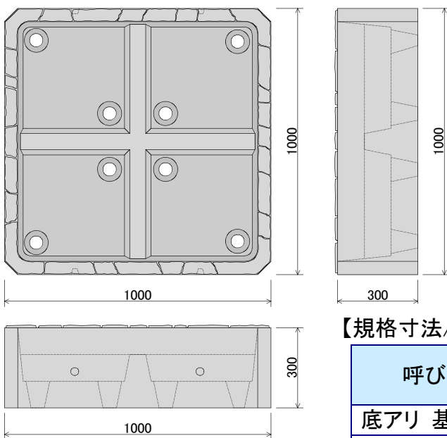
【製品図:基本型/ I型】
