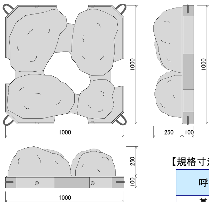
【製品図：基本型】
